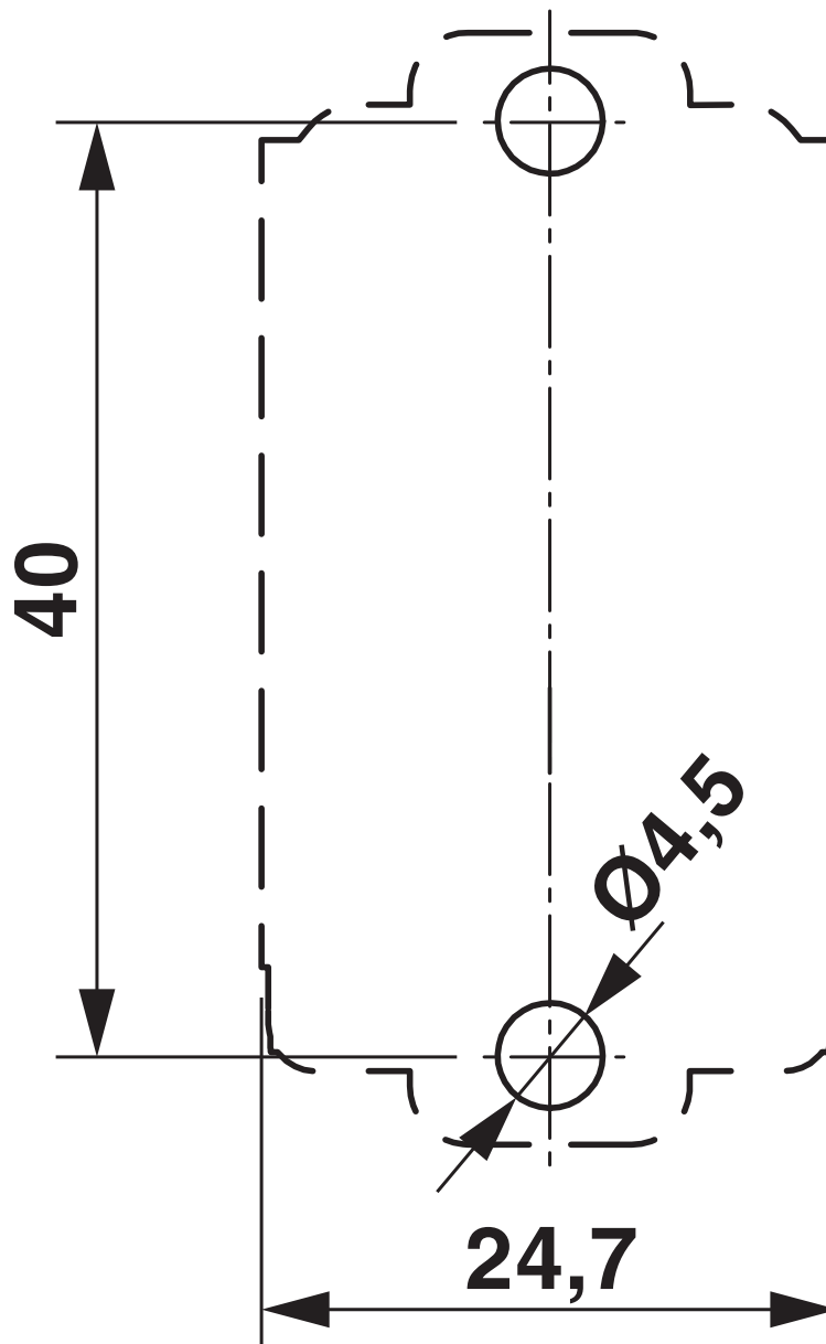
Bohrplan/Lötpadgeometrie
