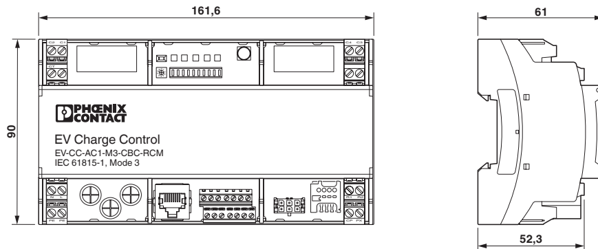
Maßzeichnung
