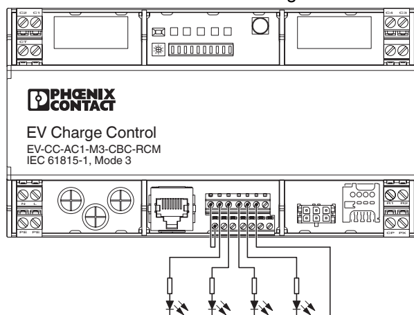
Anschlusszeichnung
