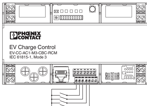
Anschlusszeichnung
