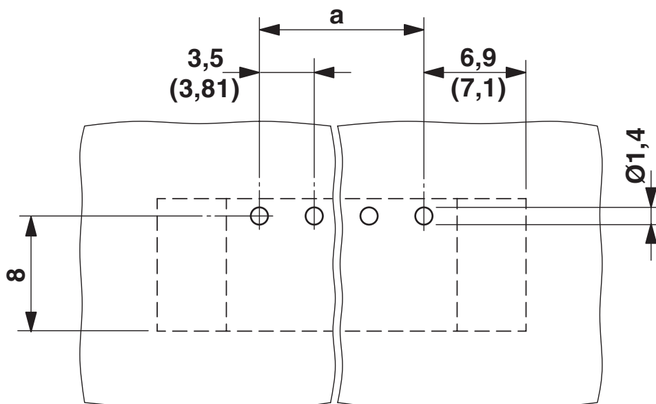
Bohrplan/Lötpadgeometrie
