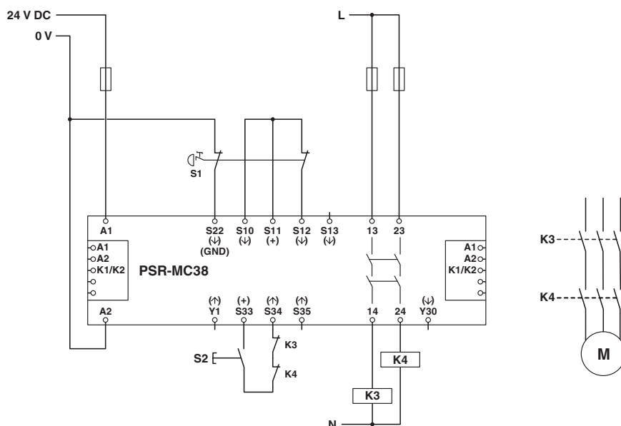
Schaltplan
