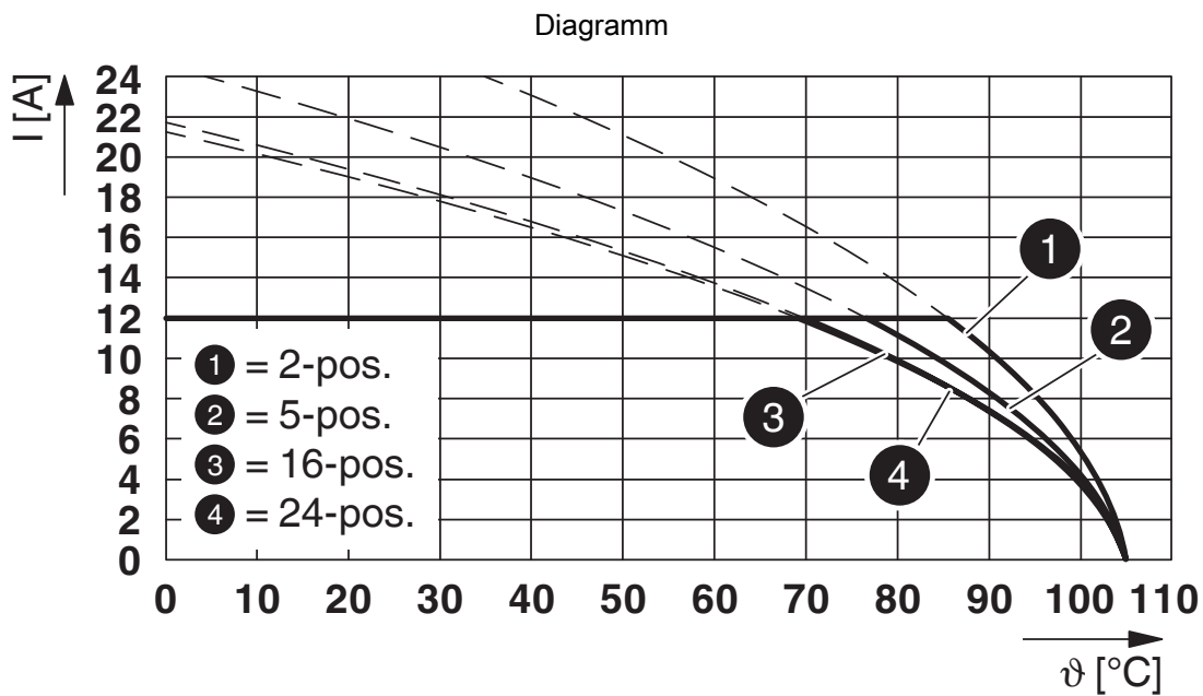
Typ: FKCOR 2,5/...-ST-5,08 mit MSTB 2,5/...-G-5,08
