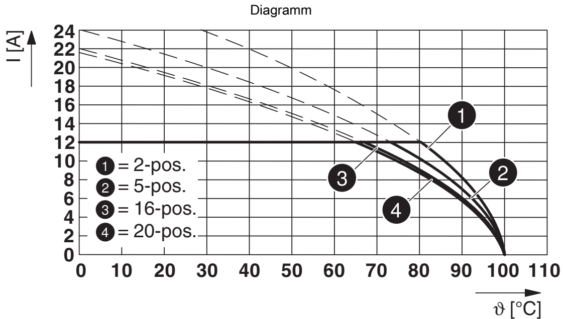
Typ: FKCT 2,5/...-ST-5,08 mit MSTB 2,5/...-G-5,08
