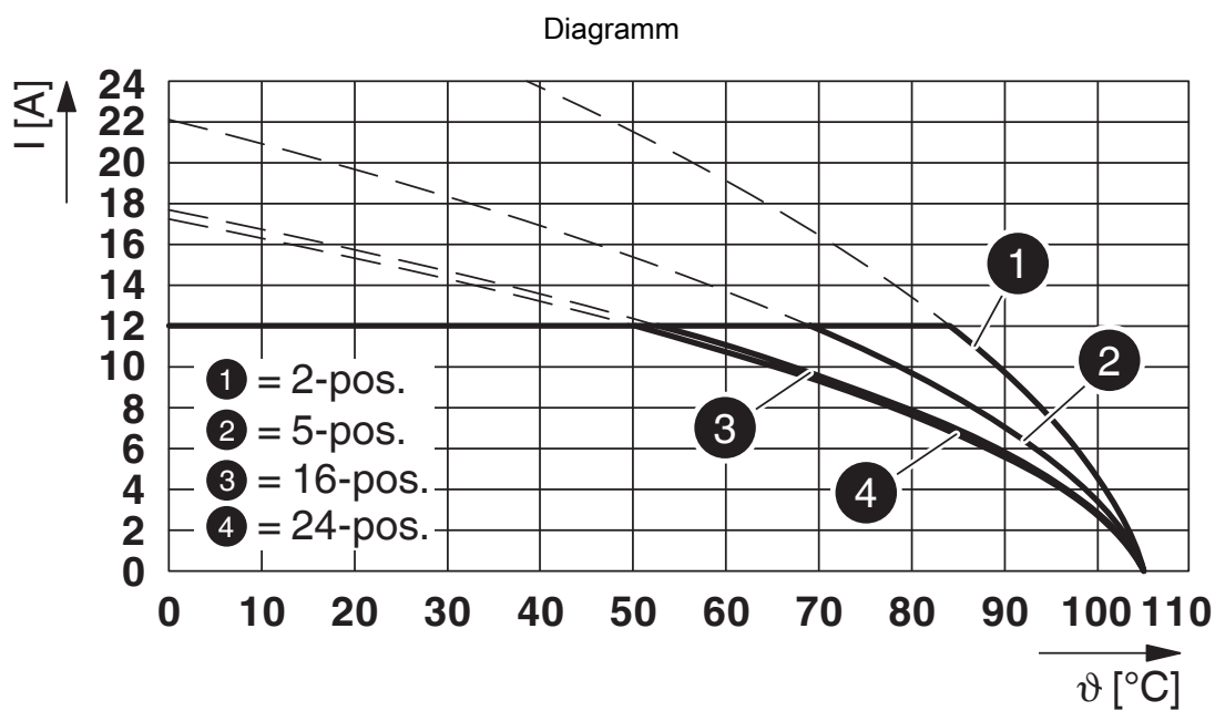
Typ: ICV 2,5/...-G-5,08 mit MSTB 2,5/...-G-5,08
