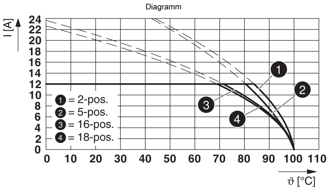
Typ: FKCN 2,5/...-ST-5,08 mit MSTB 2,5/...-G-5,08
