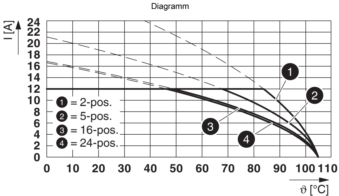
Typ: IC 2,5/...-G-5,08 mit MSTB 2,5/...-G-5,08
