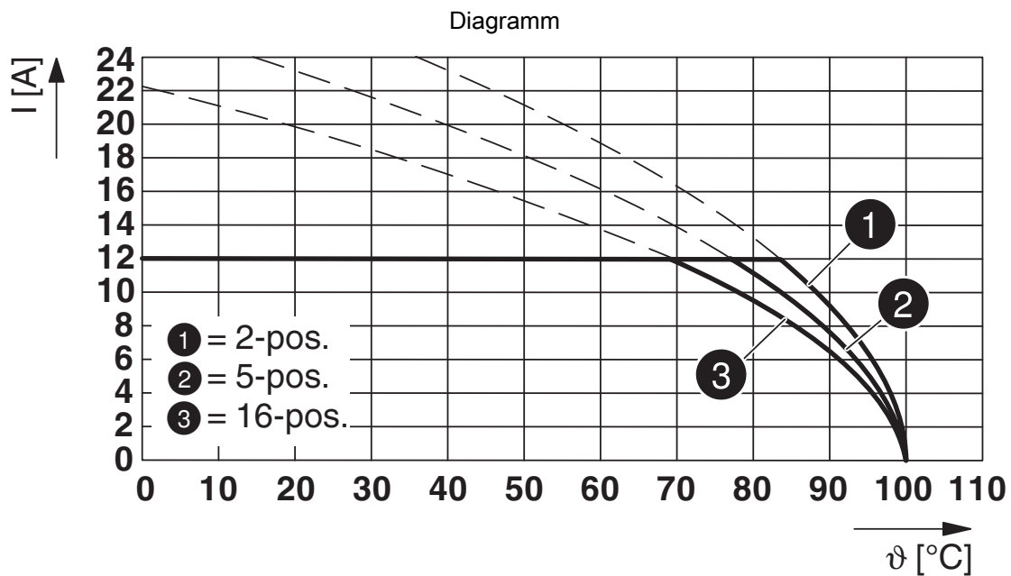
Typ: FKCV(W/R) 2,5/...-ST-5,08 mit MSTB 2,5/...-G-5,08
