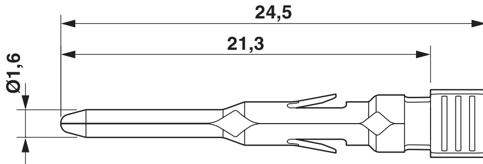
Maßzeichnung
