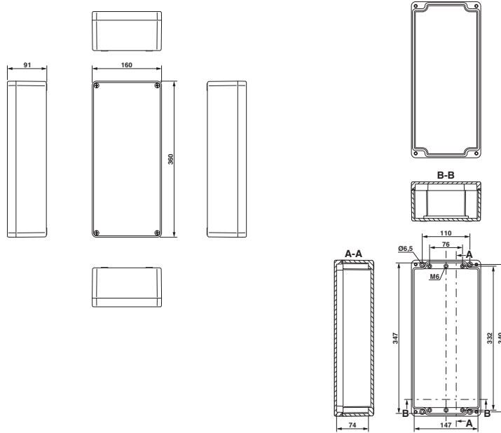
Schemazeichnung
