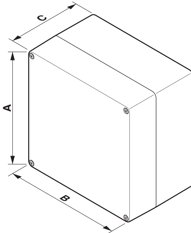
Schemazeichnung
