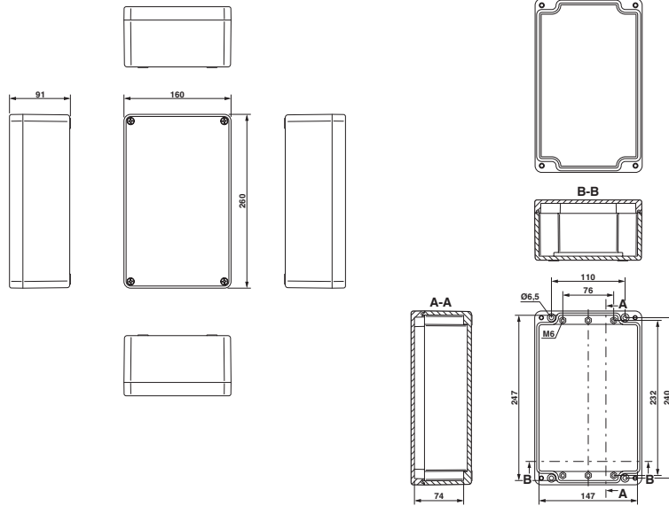
Schemazeichnung
