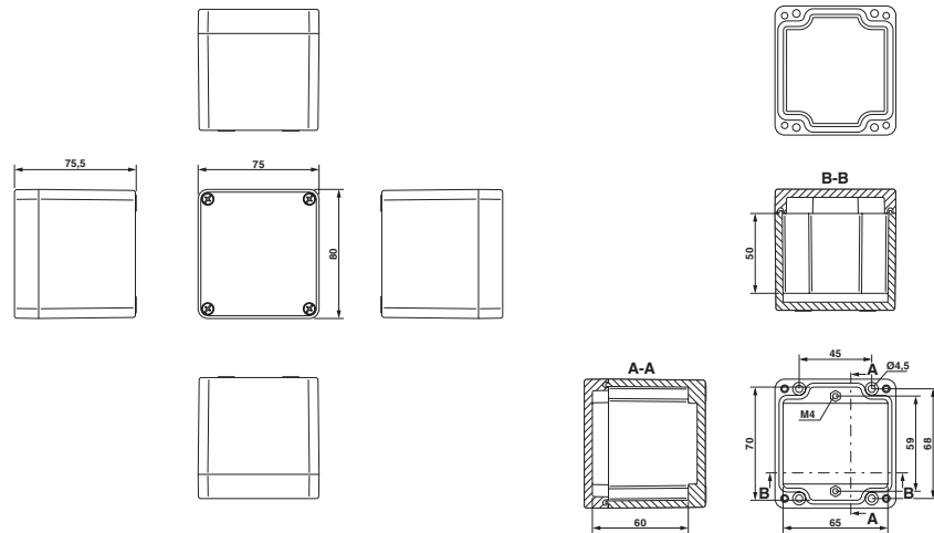
Maßzeichnung
