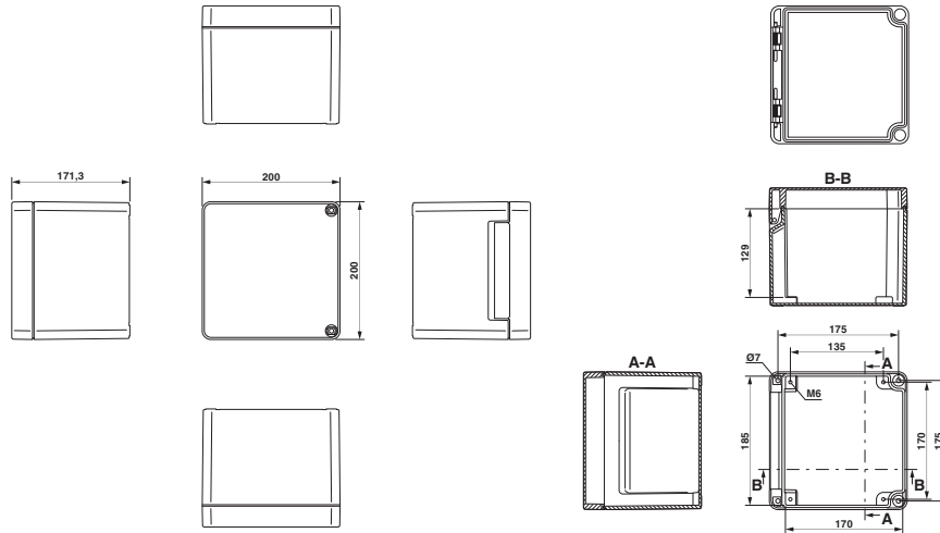
Maßzeichnung
