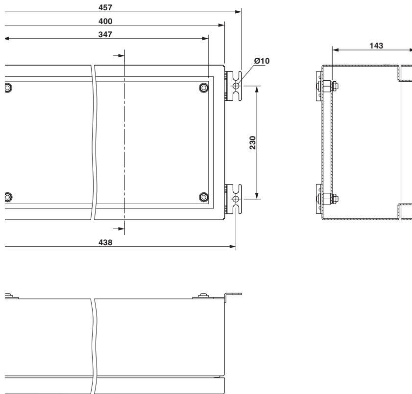
Maßzeichnung
