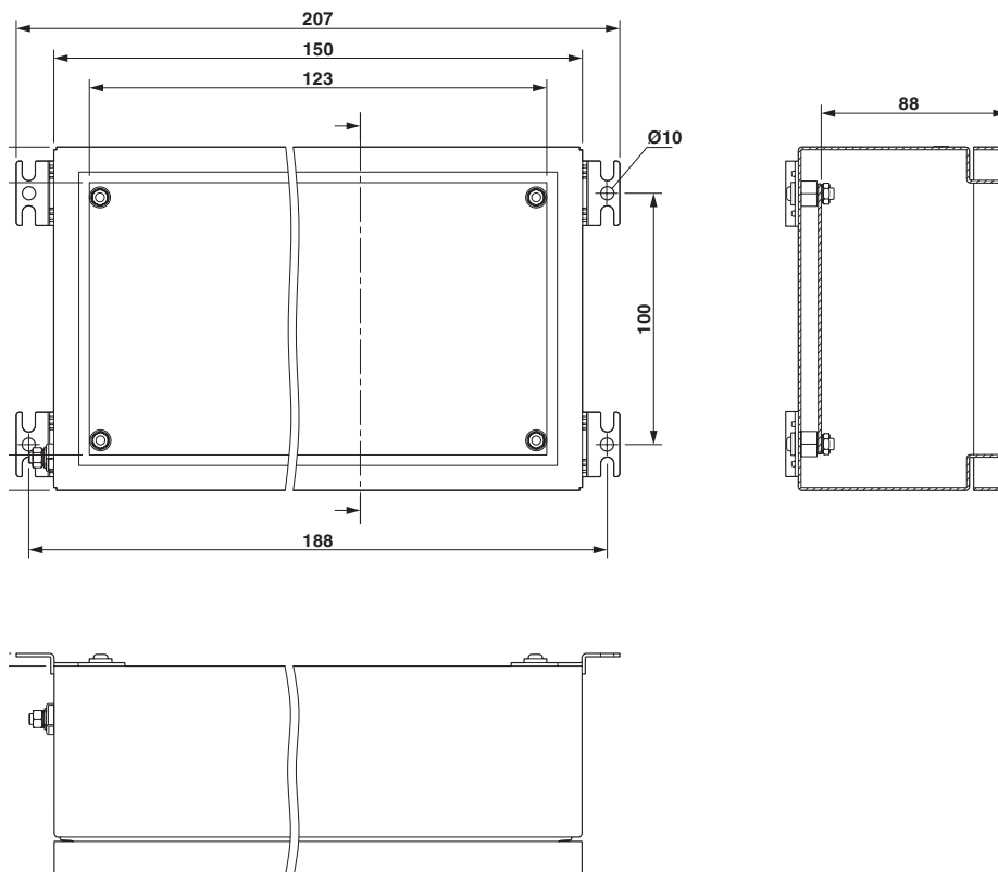
Maßzeichnung
