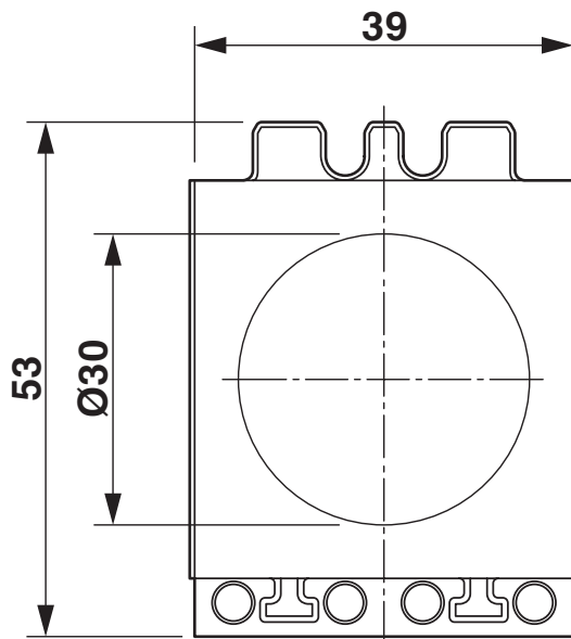
Maßzeichnung
