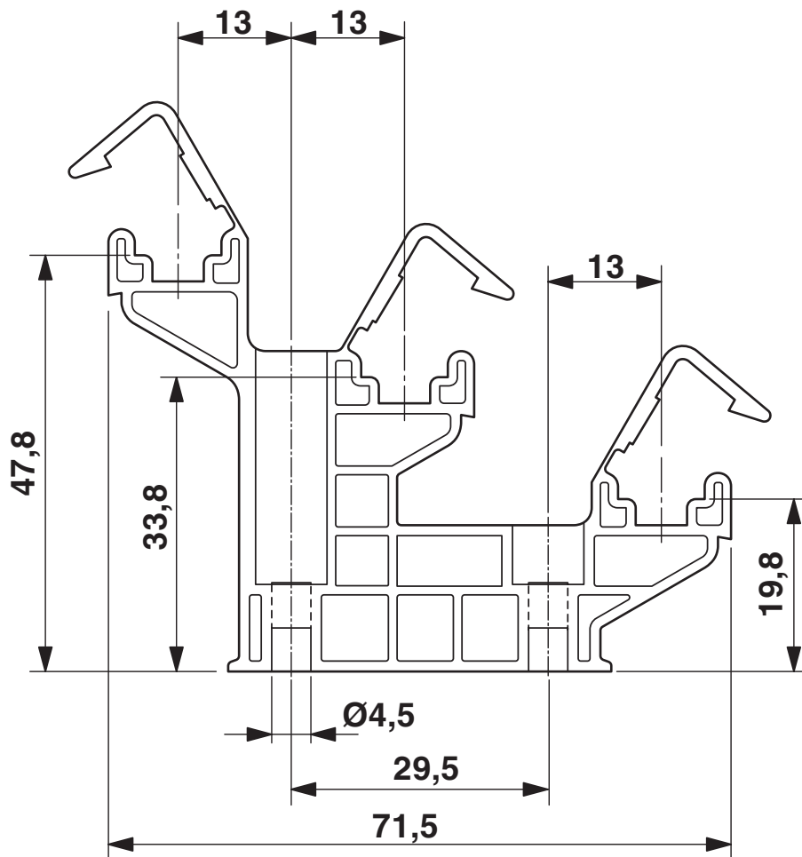
Maßzeichnung
