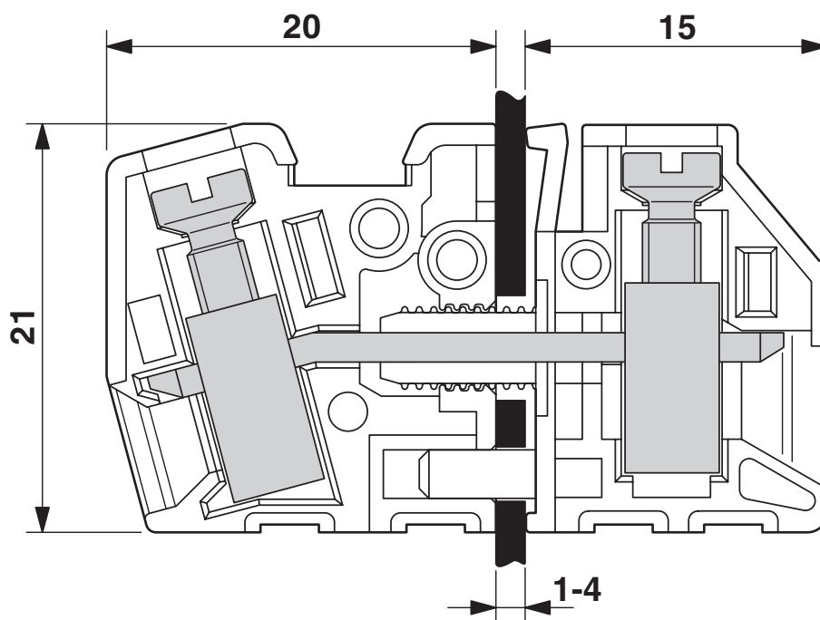
Maßzeichnung
