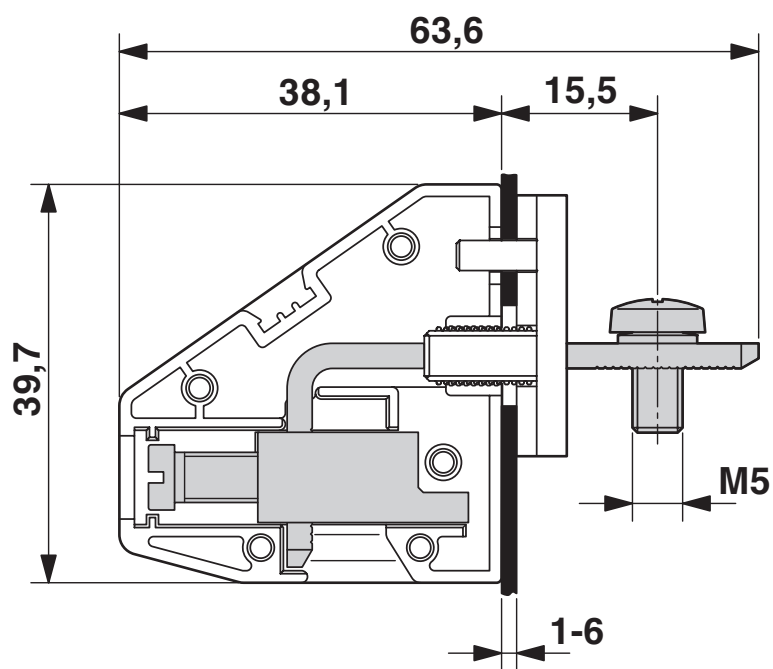
Maßzeichnung
