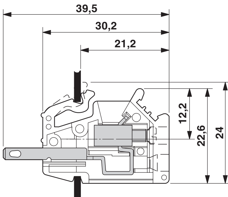
Maßzeichnung
