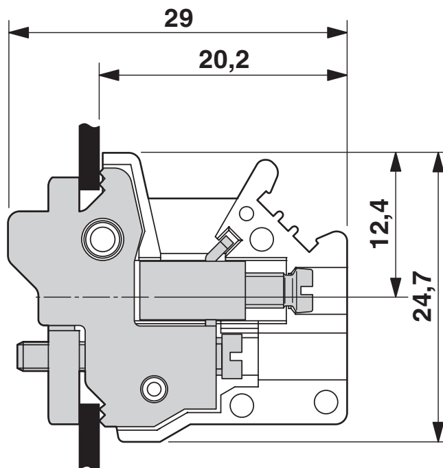
Maßzeichnung
