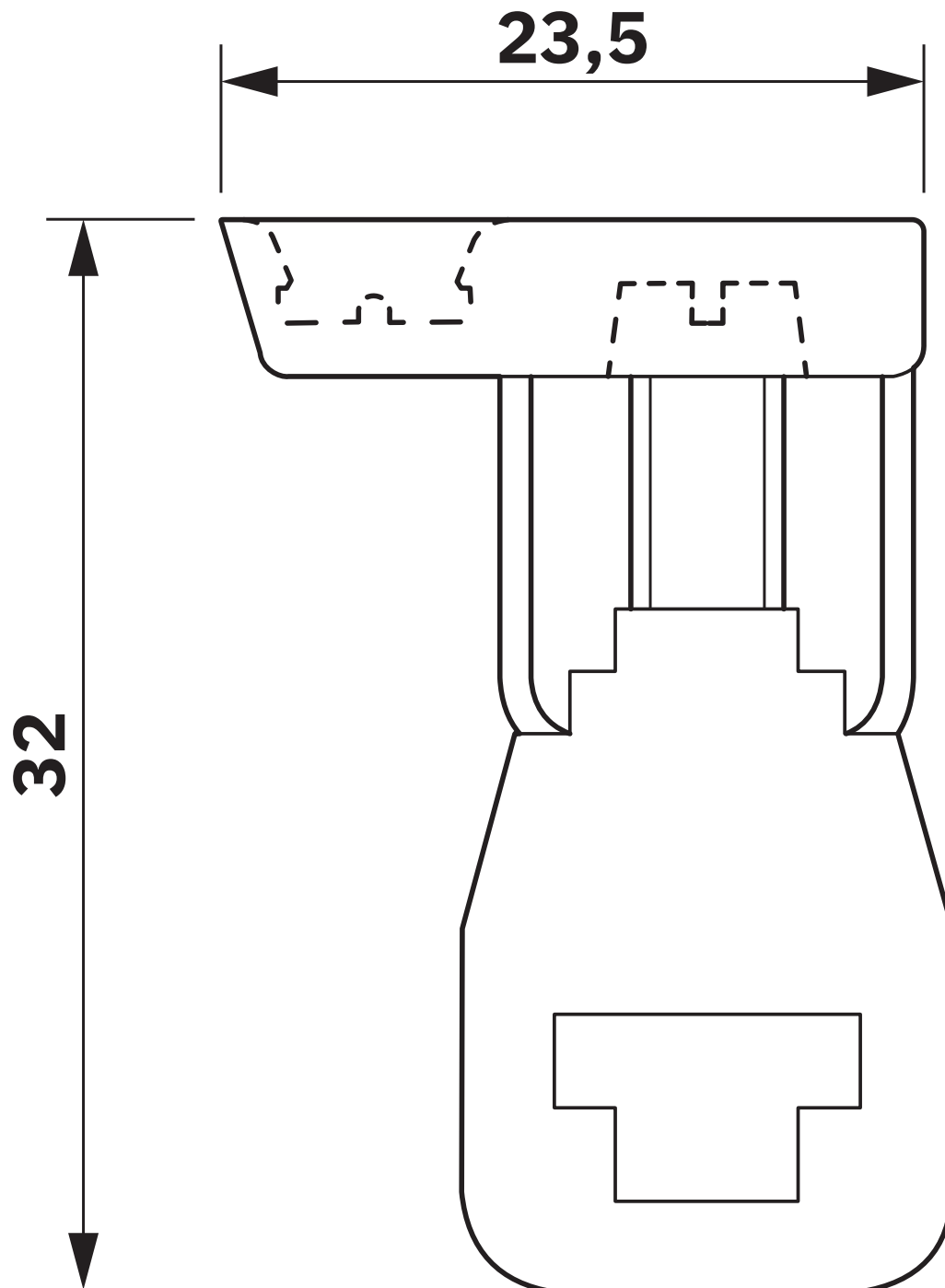
Maßzeichnung
