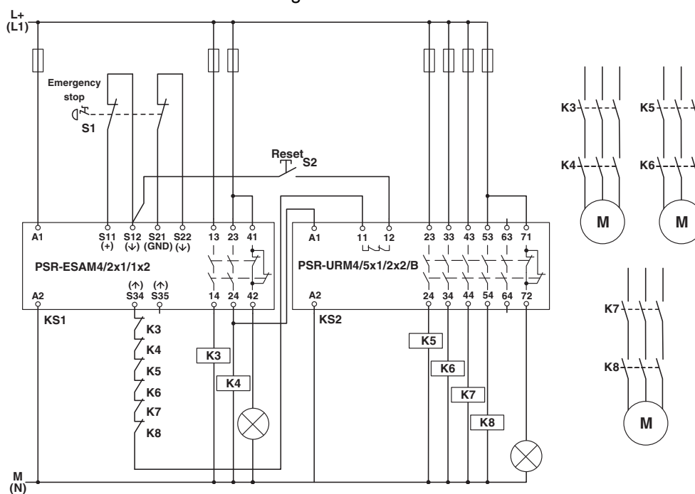
Monitoramento de parada de emergência de dois canais com expansão de contato
