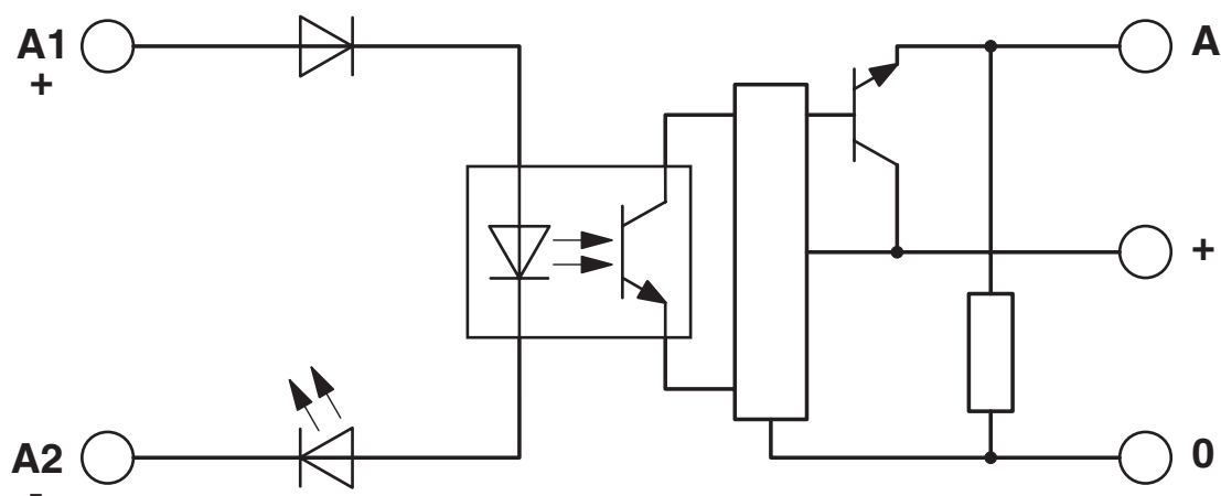
Diagrama de circuitos
