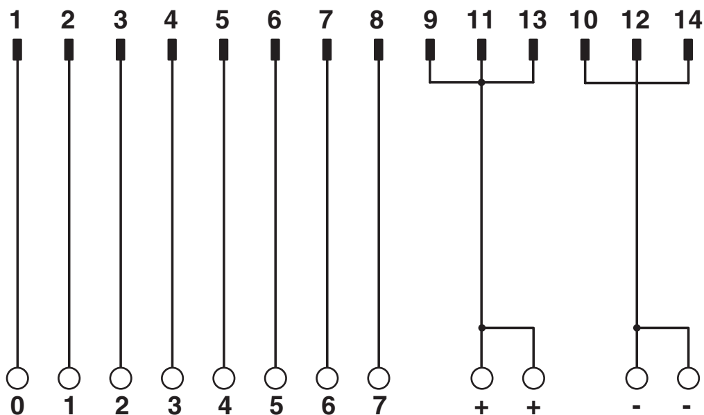
Diagrama de conexões UM 45-FLK14/PLC
