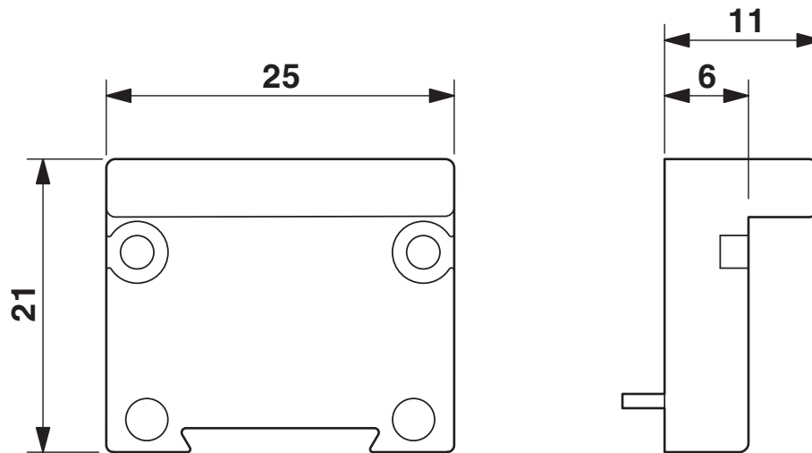
Desenho de medidas
