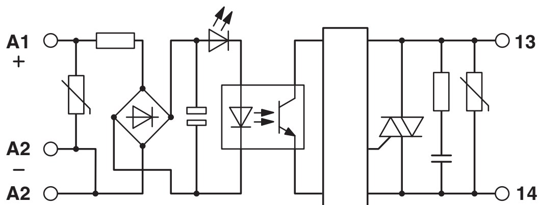
Diagrama de circuitos
