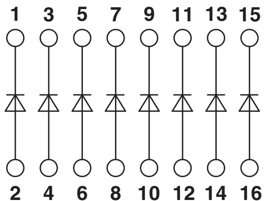
Diagrama de circuitos
