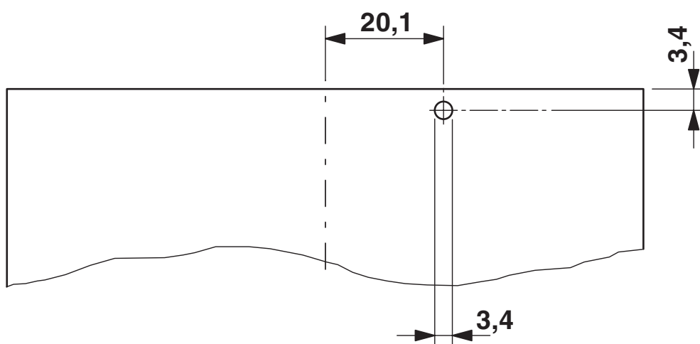
Esquema de pinagem/Geometria de pino de solda
