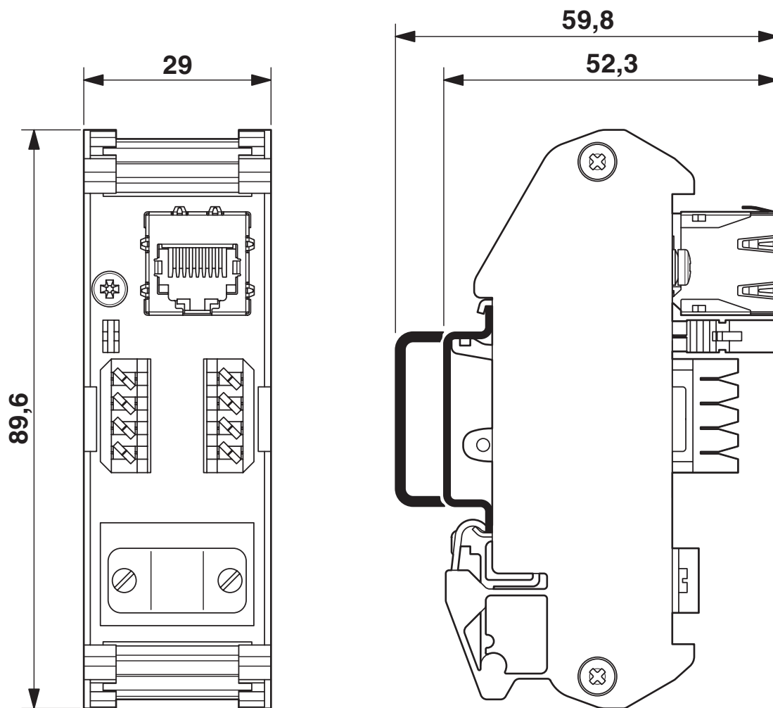
Desenho com dimensões
