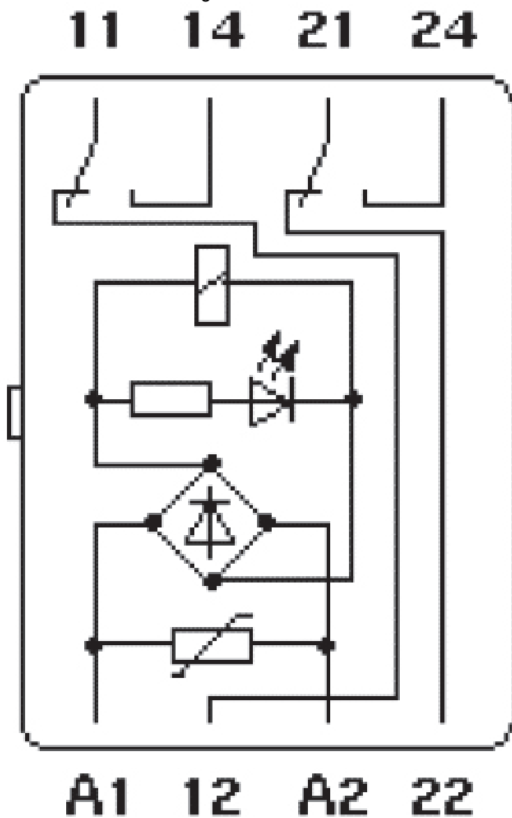
Diagrama de circuitos
