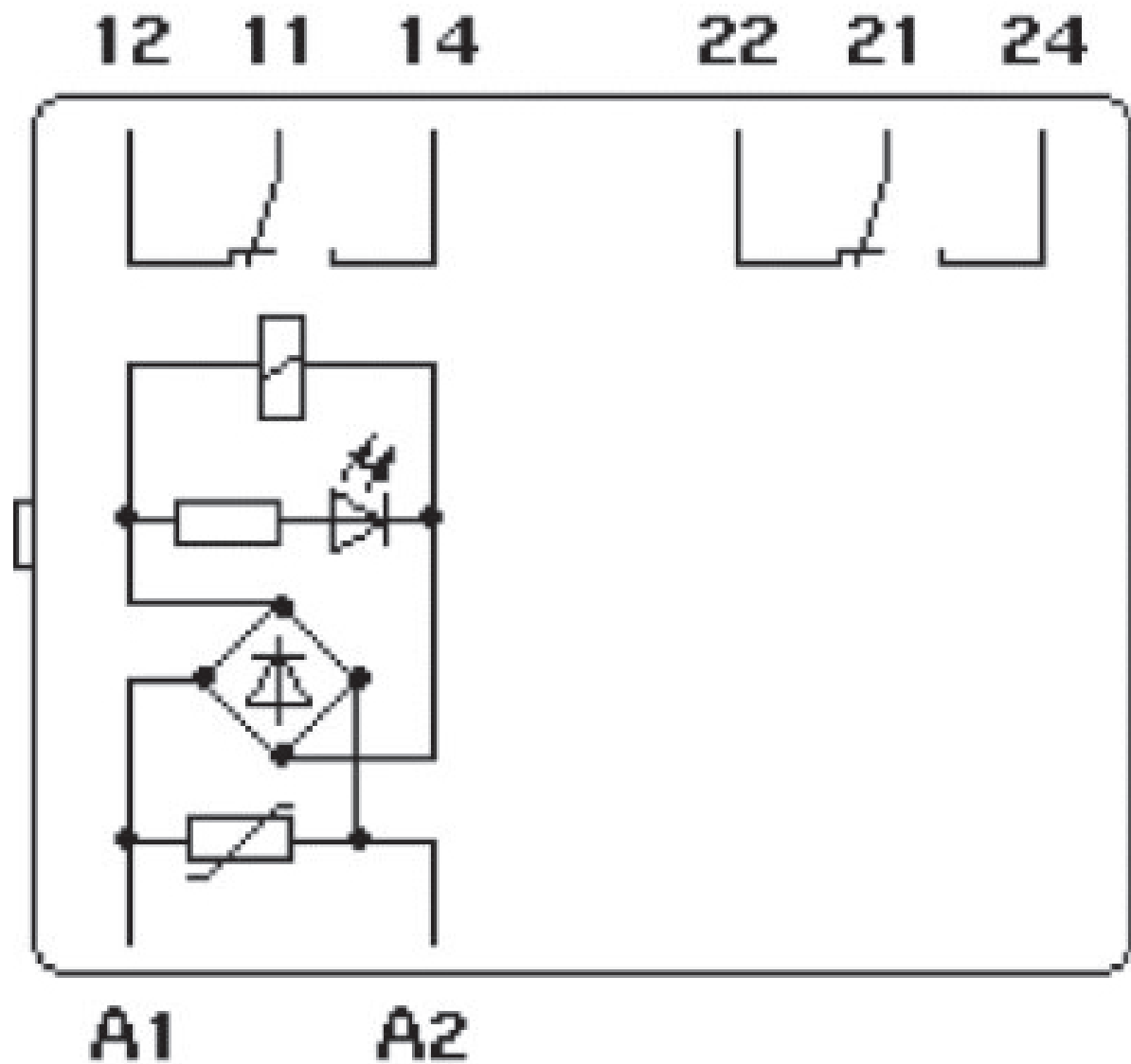
Diagrama de circuitos
