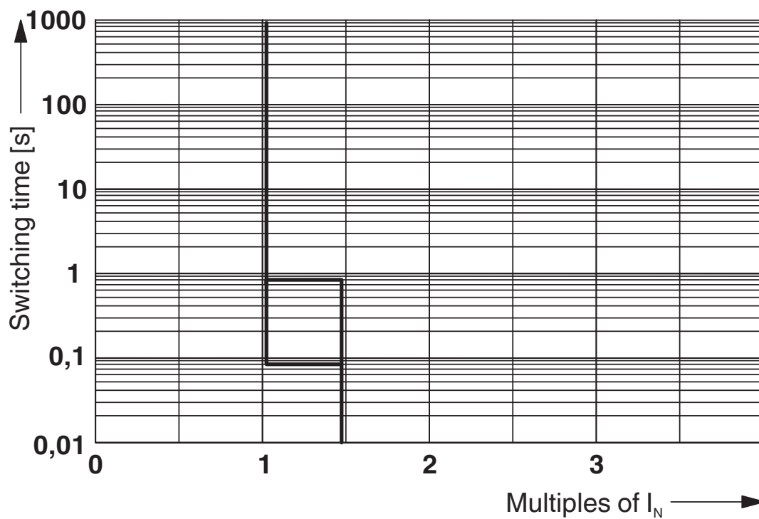
Curva característica de disparo
