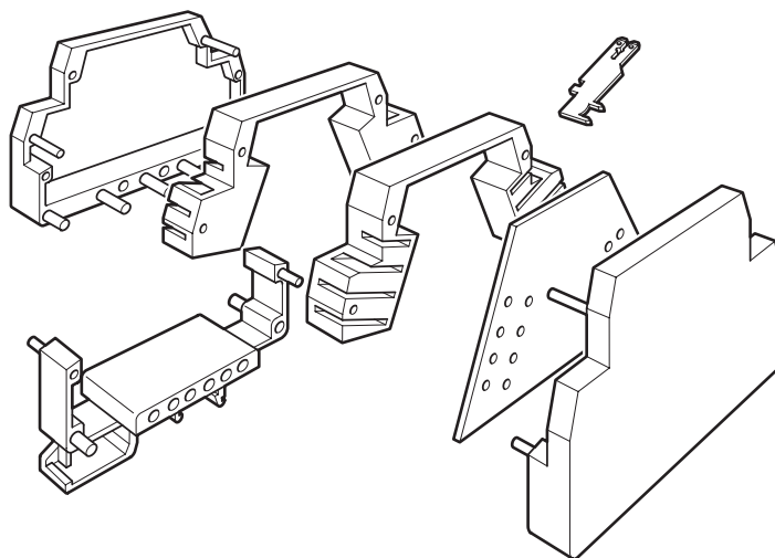
Desenho expandido
