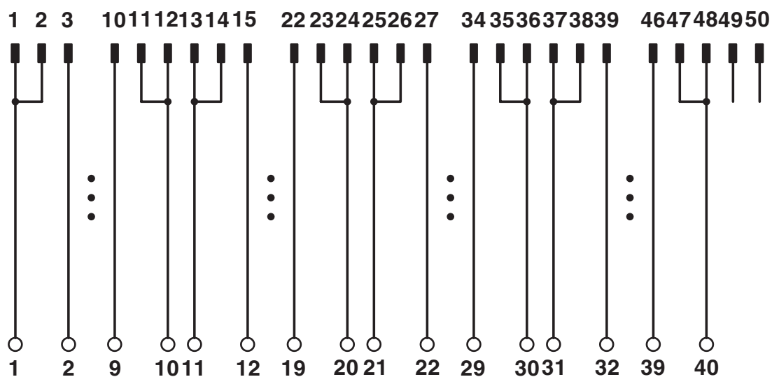
Diagrama de conexões VIP-2/.../FLK50 (1-40) /S7
