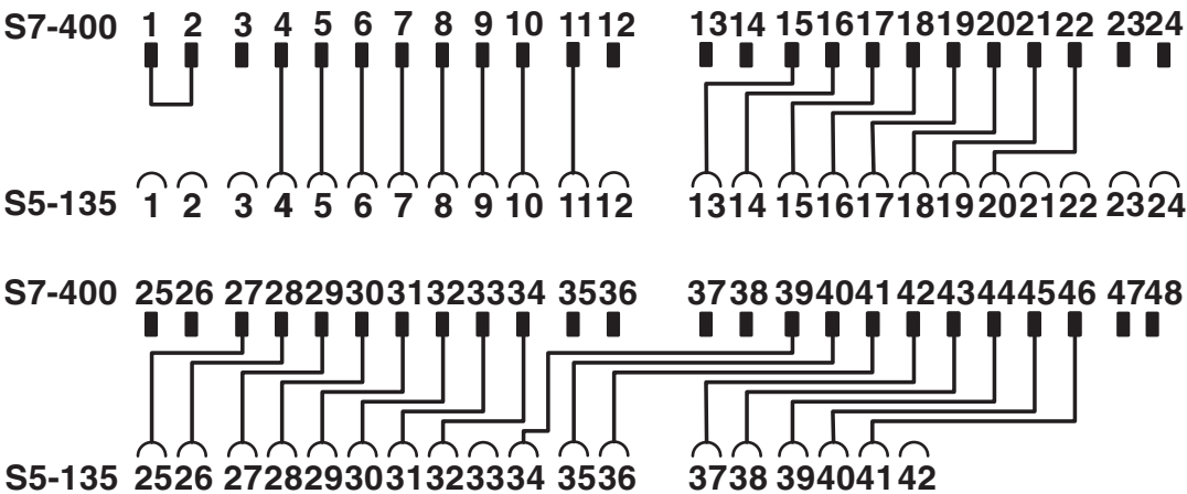
Diagrama de conexões FLKM S135-431-UA/S400
