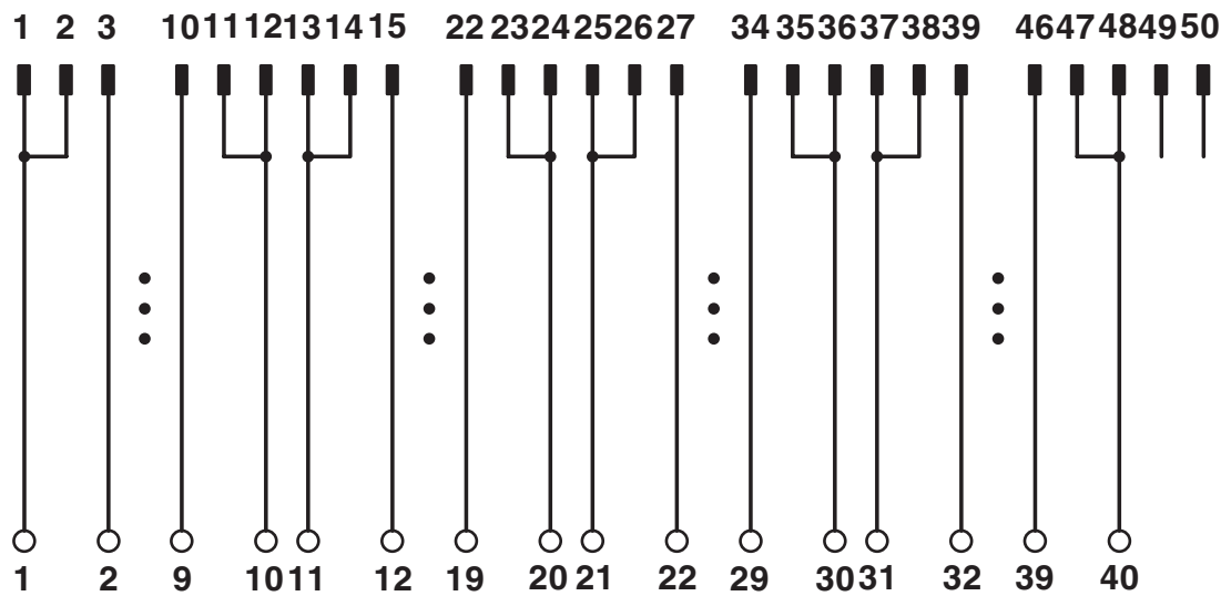
Diagrama de conexões UM 45-FLK50/S7-300
