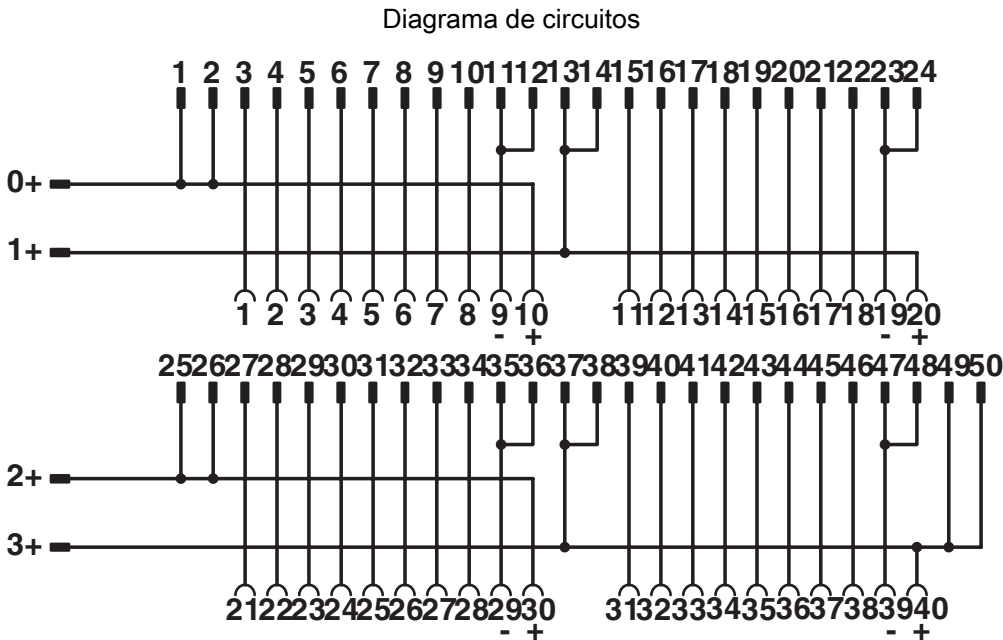
Diagrama de conexões FLKM 50-PA-MODI-TSX/Q
