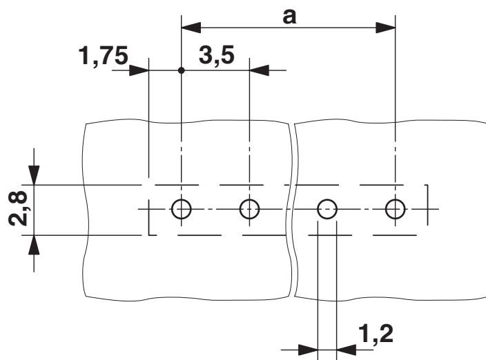
Esquema de pinagem/Geometria de pino de solda
