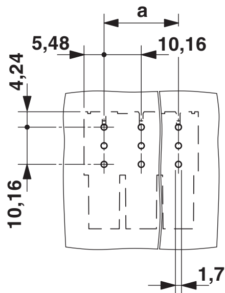
Esquema de pinagem/Geometria de pino de solda
