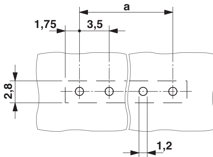
Esquema de pinagem/Geometria de pino de solda
