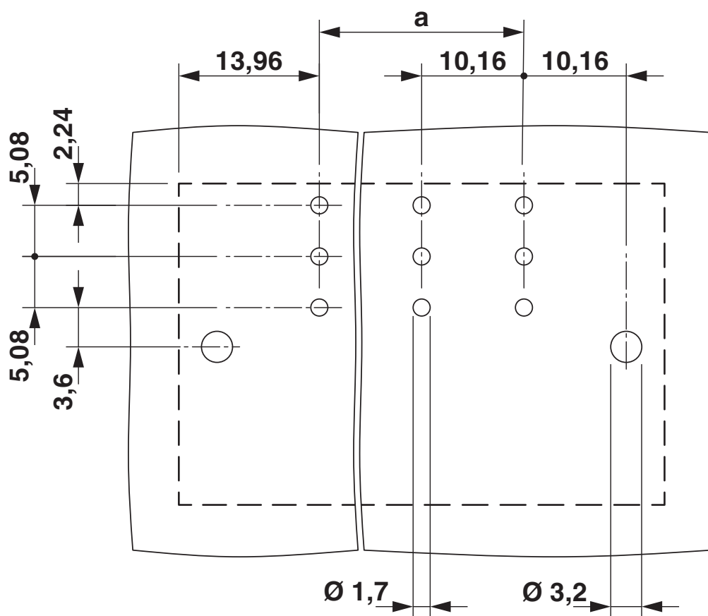
Esquema de pinagem/Geometria de pino de solda
