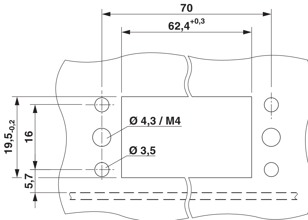
a - Placa circuito impresso
