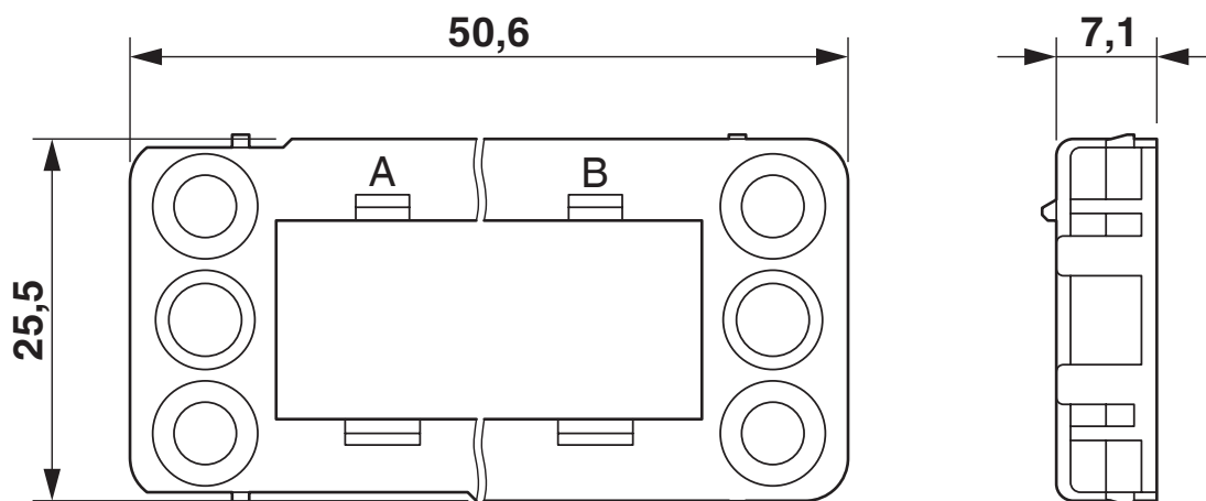
Desenho cotado, moldura de montagem
