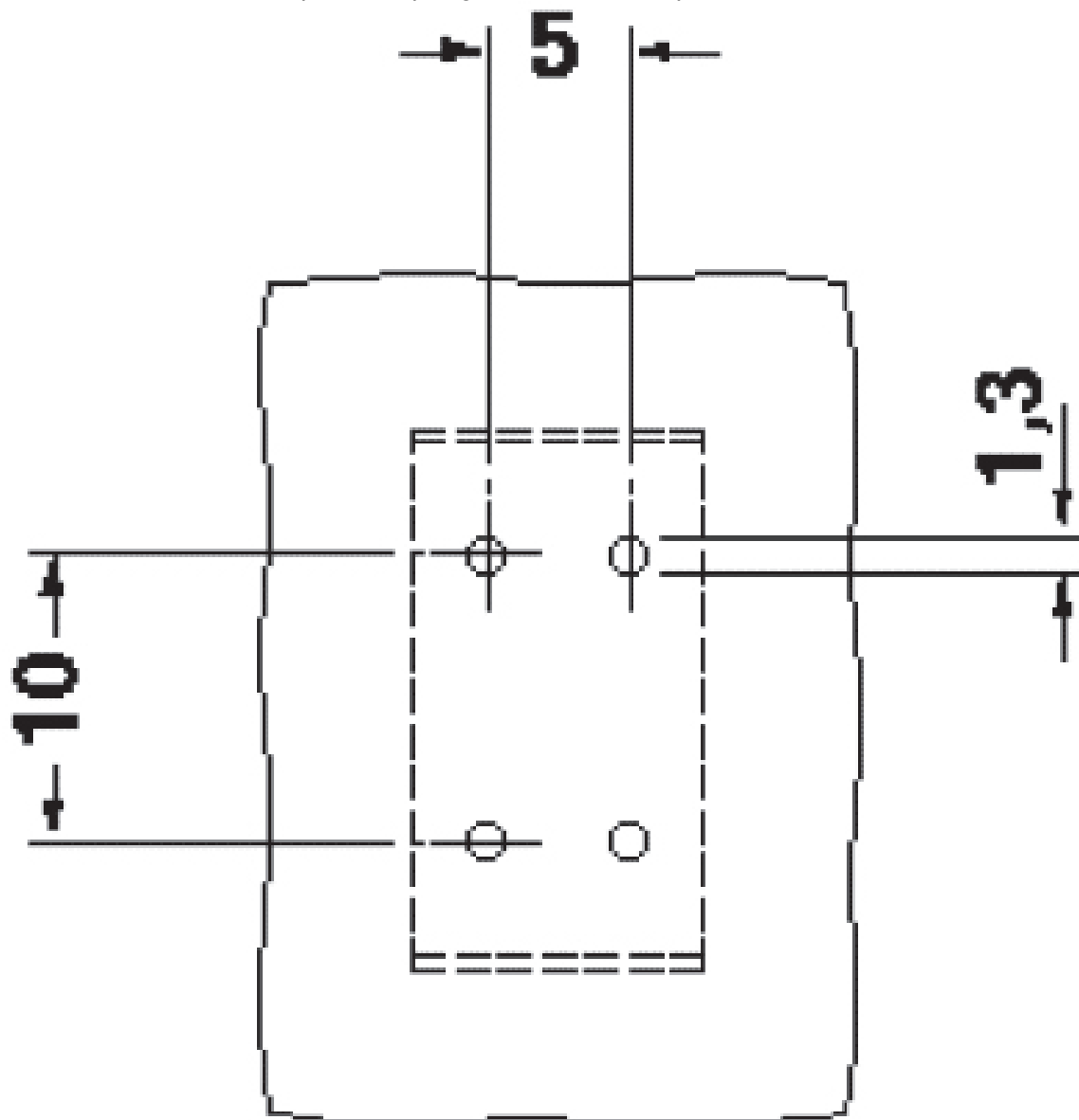
Esquema de pinagem/Geometria de pino de solda
