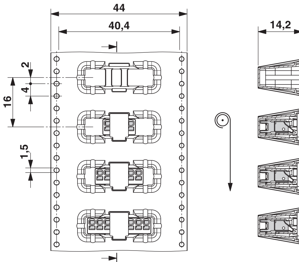
Desenho de medidas
