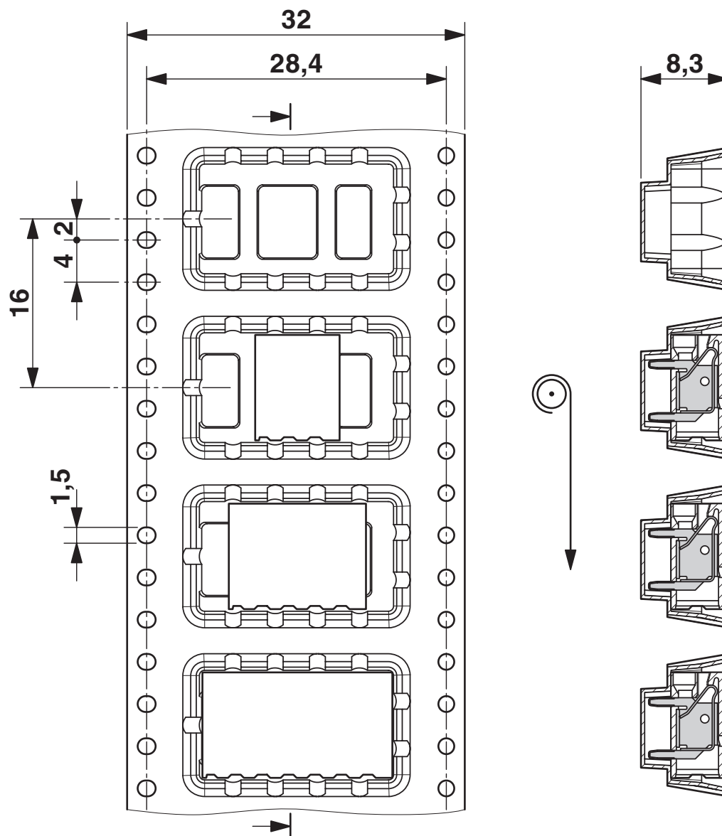
Desenho de medidas
