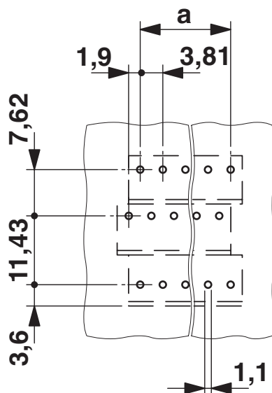
Esquema de pinagem/Geometria de pino de solda
