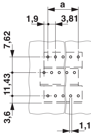
Esquema de pinagem/Geometria de pino de solda
