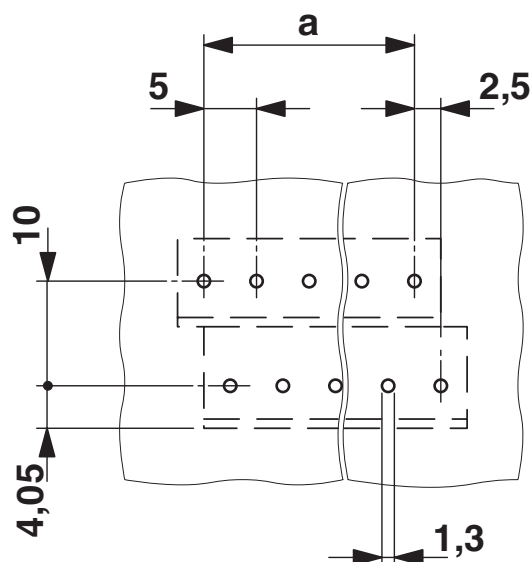
Esquema de pinagem/Geometria de pino de solda
