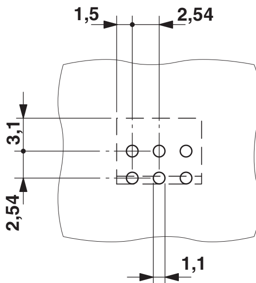
Esquema de pinagem/Geometria de pino de solda
