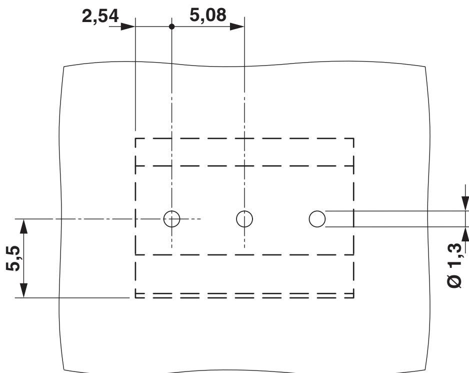
Esquema de pinagem/Geometria de pino de solda
