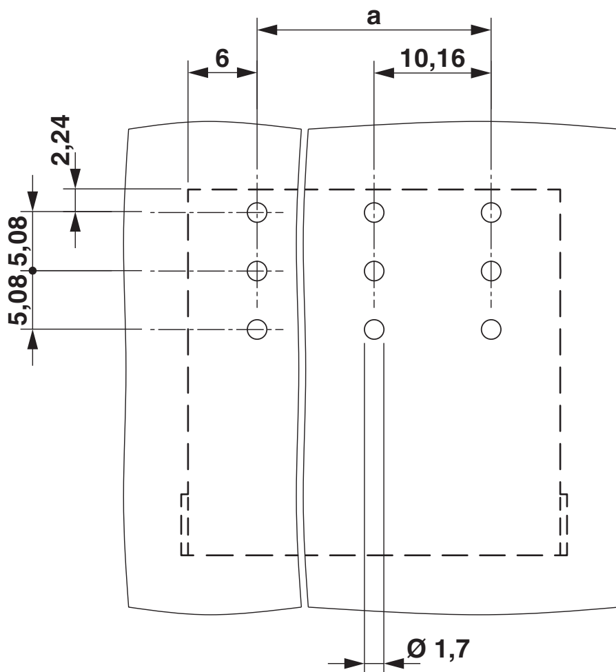
Esquema de pinagem/Geometria de pino de solda
